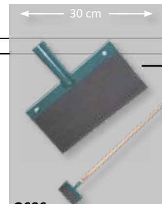
G686 RACLOIR DE COFFREUR Lame en acier boulonnée avec manche en bois frêne poncé ciré 1,20 m
