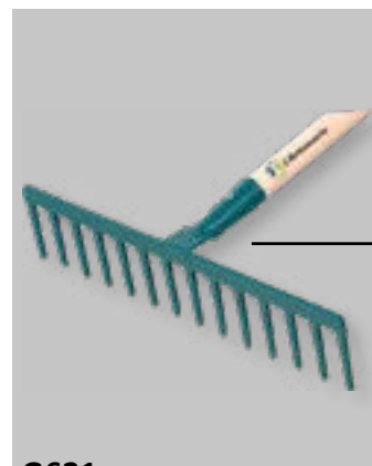
G621 RATEAU FORGÉ 14 DENTS DROITES 40 CM Manche bois frêne poncé ciré 1,50 m. Douille forgée
